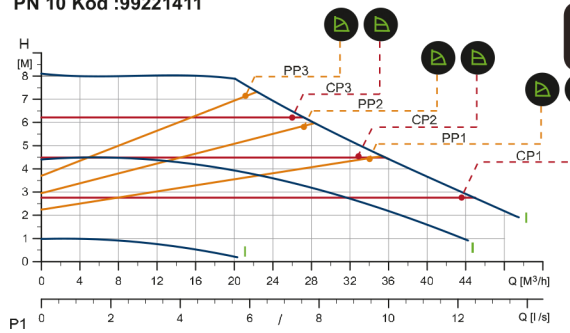
MAGNA 1 80-80 F 1 x 230 V, 50/60 Hz PN 6 Kod :99221407 PN 10 Kod :99221411
