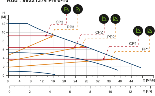
MAGNA 1 65-120 F 1 x 230 V, 50/60 Hz Kod : 99221374 PN 6-10
