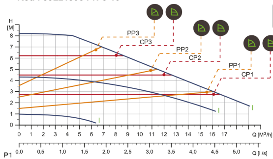
MAGNA 1 40-80 F 1 x 230 V, 50/60 Hz Kod : 99221303 PN 6-10
