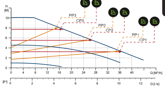
MAGNA 1 65-100 F 1 x 230 V, 50/60 Hz Kod : 99221373 PN 6-10
