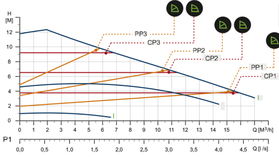
MAGNA 1 32-120 F 1 x 230 V, 50/60 Hz F.Kod : 99221285 PN 6-10
