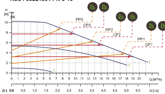
MAGNA 1 40-100 F 1 x 230 V, 50/60 Hz Kod : 99221304 PN 6-10
