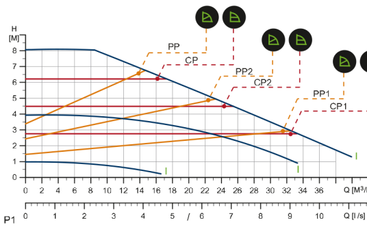
MAGNA 1 65-80 F 1 x 230 V, 50/60 Hz Kod : 99221372 PN 6-10
