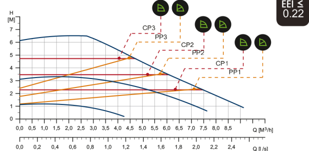
MAGNA 1 32-60 F 1 x 230 V, 50/60 Hz D.Kod : D.99221234 PN 10 F.Kod : F.99221269 PN 6-10
