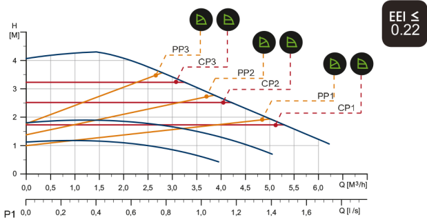
MAGNA 1 25-40 F 1 x 230 V, 50/60 Hz Kod : 99221216 PN-10
