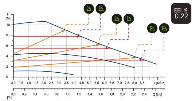
MAGNA 1 25-100 1 x 230 V, 50/60 Hz Kod : 99221214 PN-10
