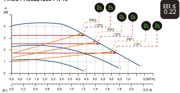
MAGNA 1 32-40 1 x 230 V, 50/60 Hz D.Kod : D.99221233 PN 6-10 F.Kod : F.99221263 PN 10
