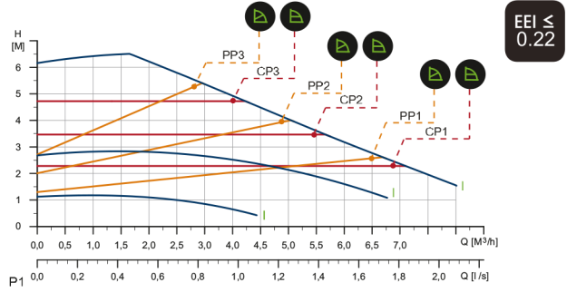
MAGNA 1 25-60 1 x 230 V, 50/60 Hz Kod : 99221217 PN-10
