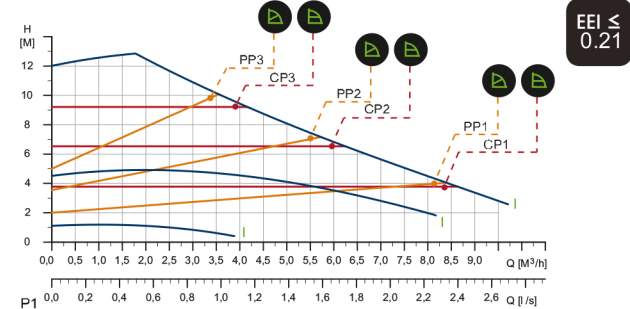
MAGNA 1 25-120 1 x 230 V, 50/60 Hz Kod : 99221215 PN-10
