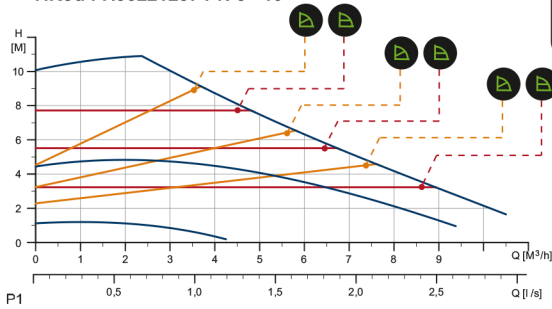
MAGNA 1 32-100 1 x 230 V, 50/60 Hz D.Kod : D.99221236 PN 10 F.Kod : F.99221237 PN 6 - 10
