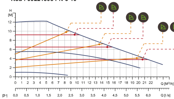
MAGNA 1 40-120 F 1 x 230 V, 50/60 Hz Kod : 99221305 PN 6-10
