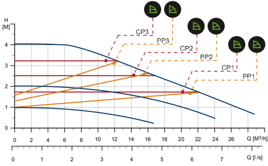
MAGNA 1 65-40 F 1 x 230 V, 50/60 Hz Kod : 99221382 PN 6-10
