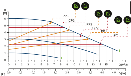
MAGNA 1 40-60 F 1 x 230 V, 50/60 Hz Kod : 99221292 PN 6-10
