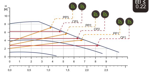
MAGNA 1 32-80 F 1 x 230 V, 50/60 Hz D.Kod : D.99221235 PN 10 F.Kod : F.99221275 PN 6-10
