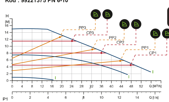
MAGNA 1 65-150 F 1 x 230 V, 50/60 Hz Kod : 99221375 PN 6-10
