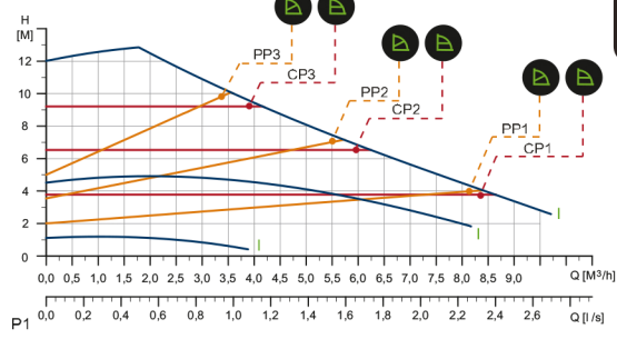
MAGNA 1 32-120 1 x 230 V, 50/60 Hz Kod : 99221281 PN 10
