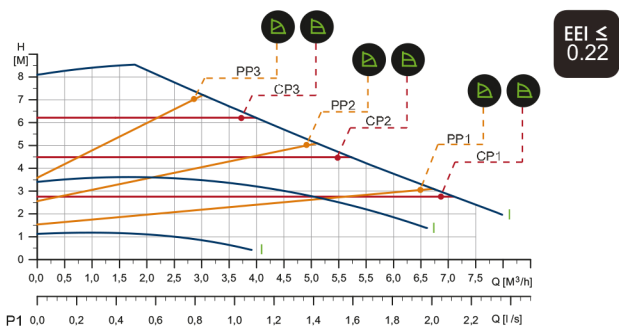
MAGNA 1 25-80 1 x 230 V, 50/60 Hz F.Kod : 99221213 PN-10
