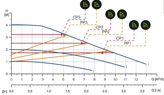
MAGNA 1 40-40 F 1 x 230 V, 50/60 Hz F.Kod : 99221291 PN 6-10
